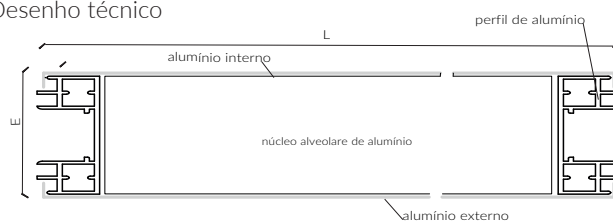
Desenho técnico
