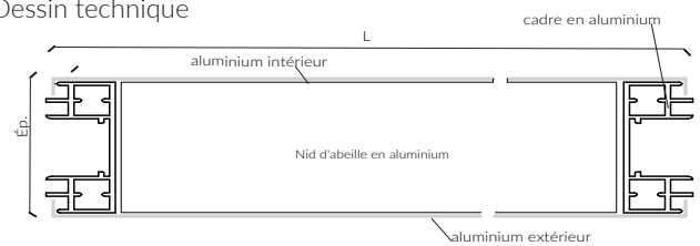
Dessin technique
