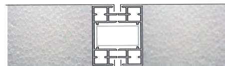
Buchse/Buchse Aluminium
