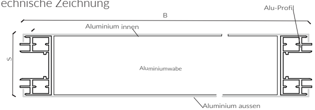
Technische Zeichnung
